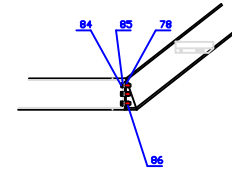
Detailansicht 'C' M 1:5
